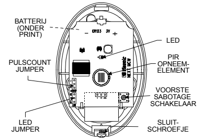
Figuur 2. Binnenwerk
