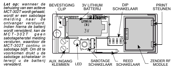
Figuur 1. MCT-302T geopend
