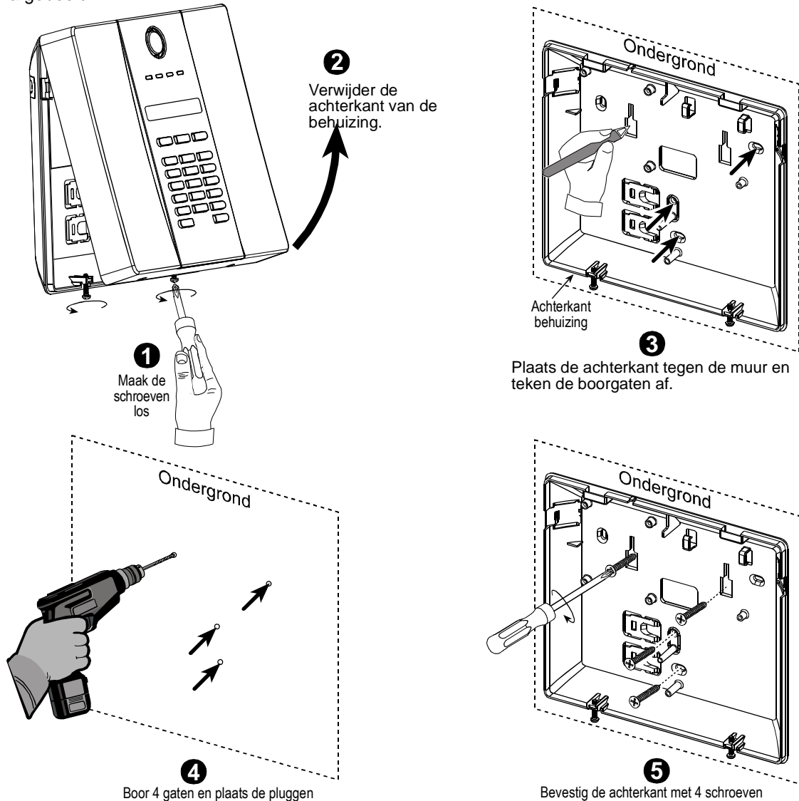
Figuur 3.1a – Montage van de achterkant van het apparaat
