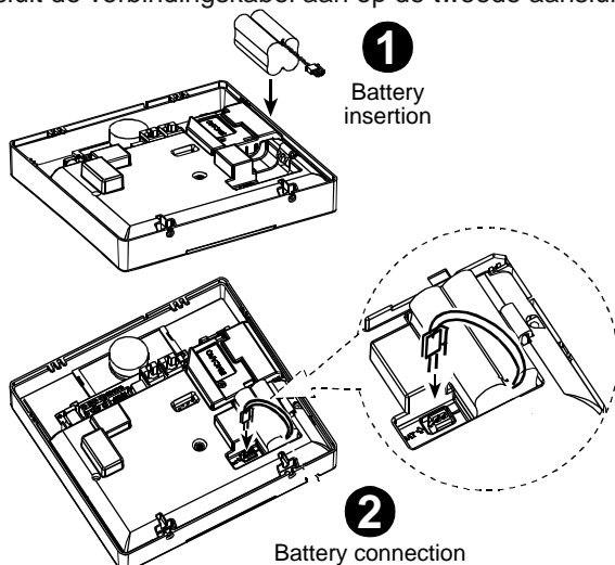
Figuur 3.1h – Batterypack plaatsen
