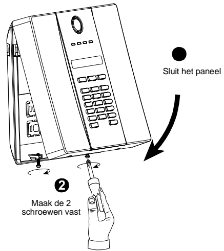
Figuur 3.1k – Behuizing sluiten
