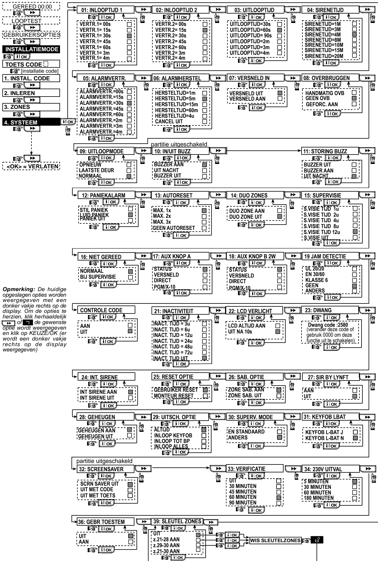
Figuur 4.4 – SYSTEEM PARAMETERS programmeerschema
