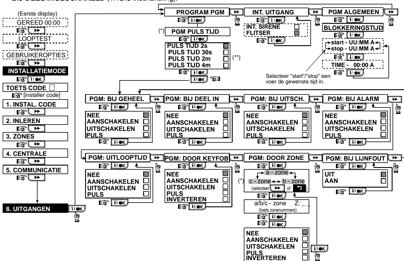
Figuur 4.8 - Definieer uitgangen Flow Chart
