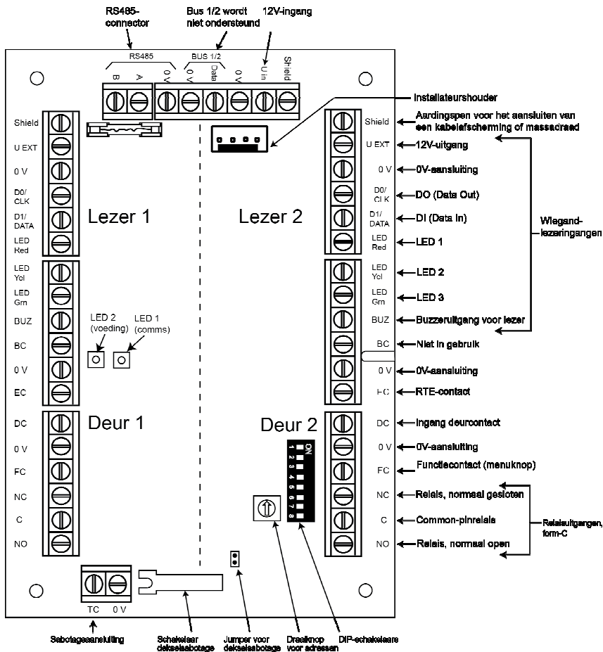
Afbeelding 17 Deurcontrolemodule PCB
