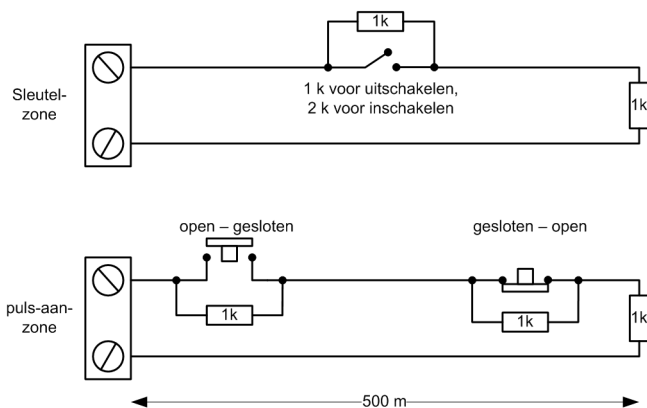
Afbeelding 7 Zonebekabeling puls-aan en sleutelschakelaar
