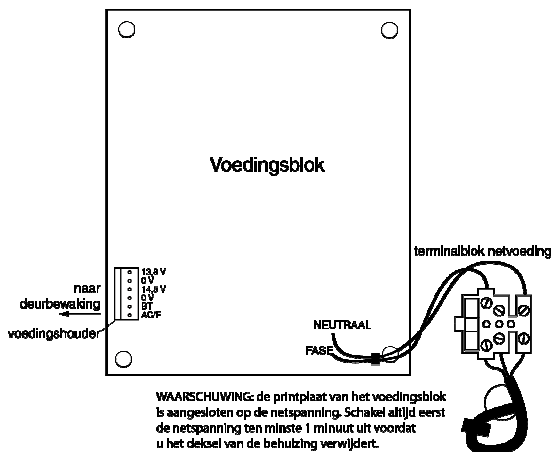
Afbeelding 14 Voedingseenheid
