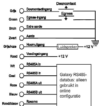
Abbeelding 13 Verbindingsdiagram
