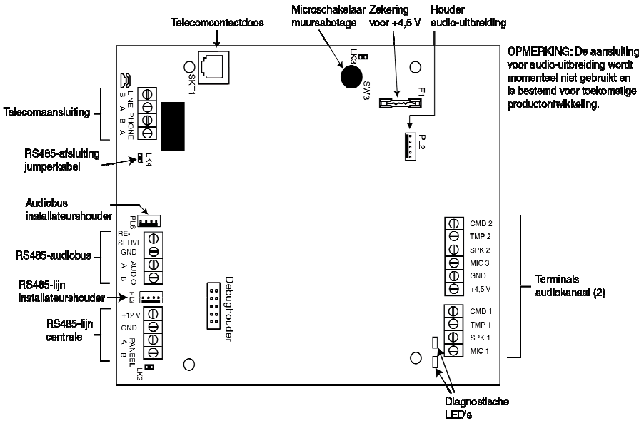
Afbeelding 15 Printplaatindeling audio-interfacemodule
