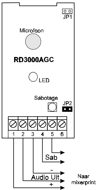
Figuur 2. Aansluiting microfoon
