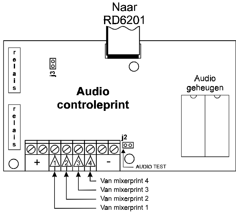
Figuur 3. Aansluiting controleprint
