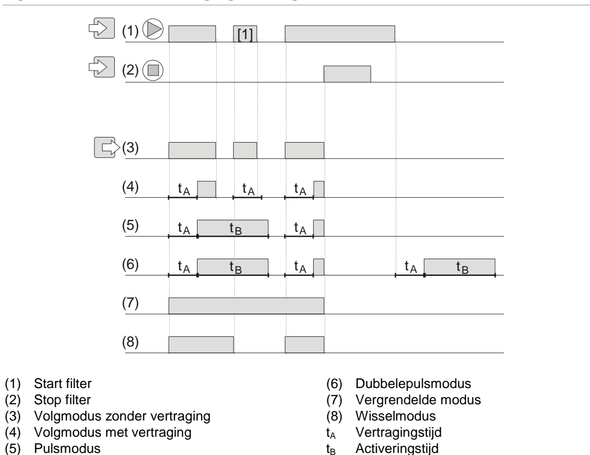
Figuur 22: Voorbeelden van uitgangactiveringsmodi
