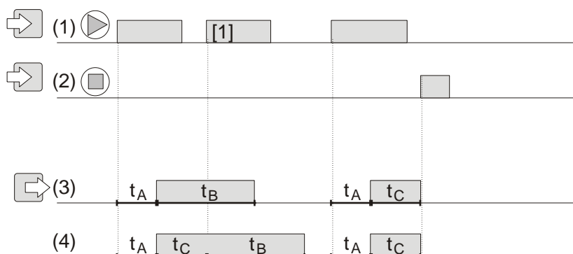
Figuur 23: Voorbeelden hertriggerbare uitgang
