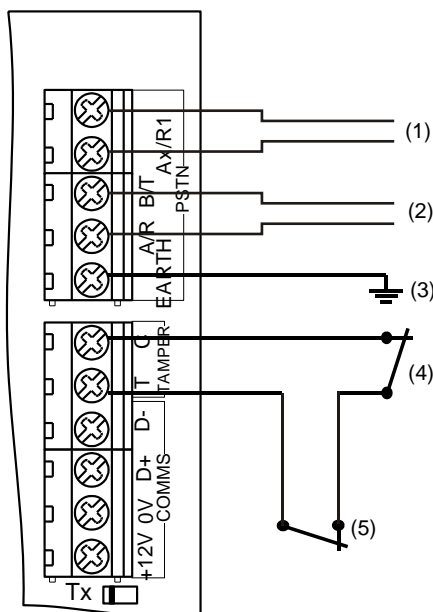
Figuur 19: Aarding, externe sabotage, en PSTN aansluiting in ATsx000A(-IP)
