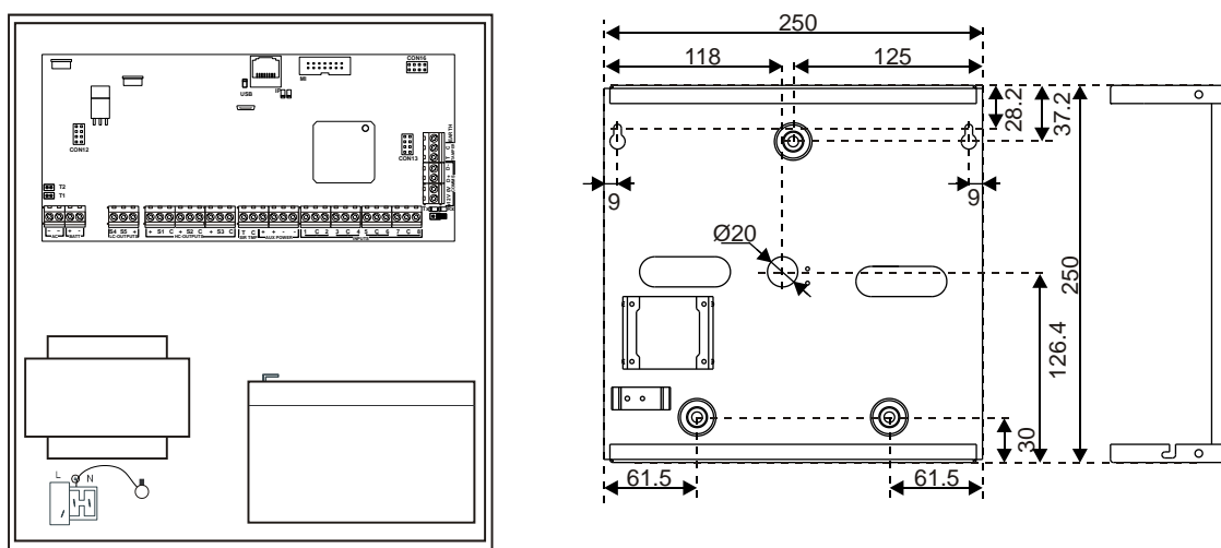
Figuur 1: Kleine metalen behuizing (-SM)
