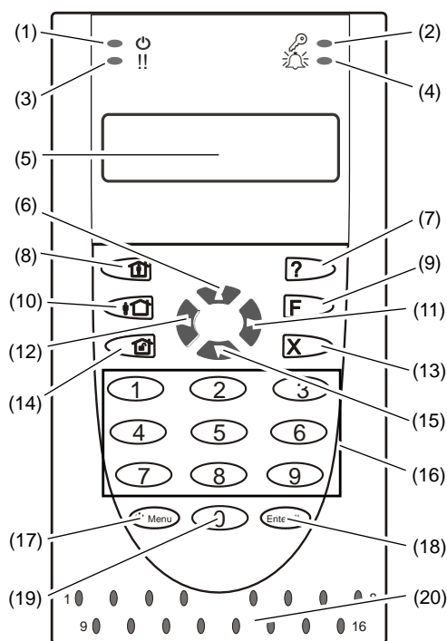
Figuur 8: ATS111xA-gebruikersinterface
