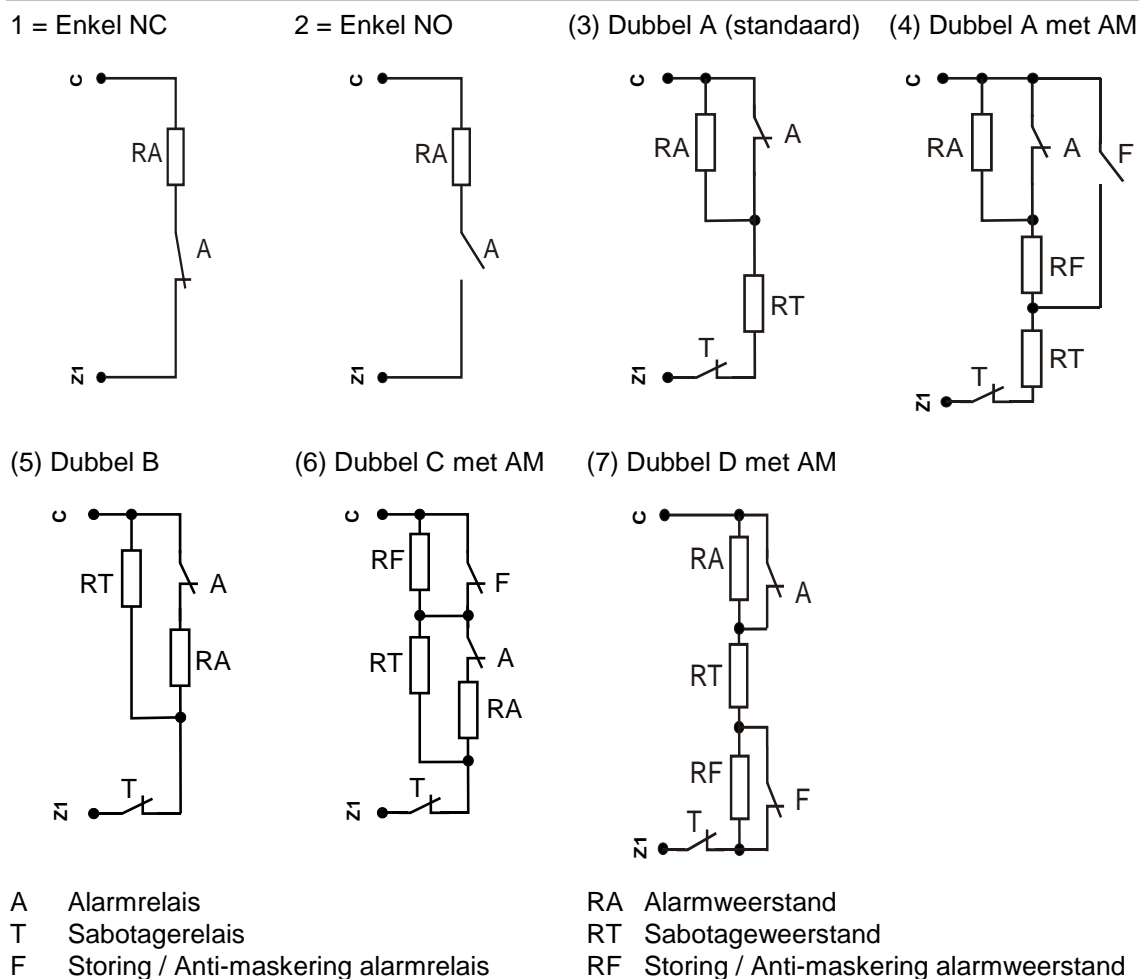
Figuur 17: Type aansluiting
