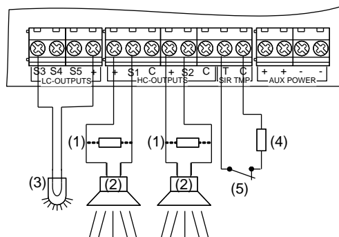
Figuur 18: Voorbeelden sirene-aansluiting
