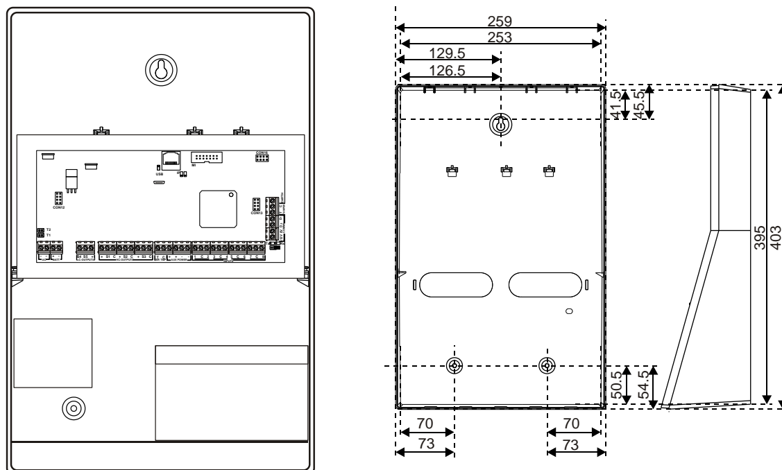
Figuur 3: Grote polycarbonaat behuizing (-LP)
