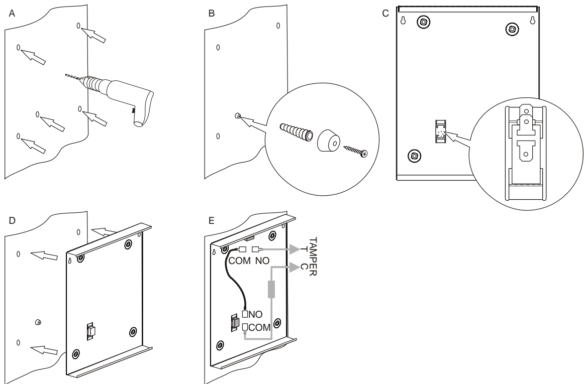
Figuur 6: Montage normale (-MM) behuizing afneembeveiliging
