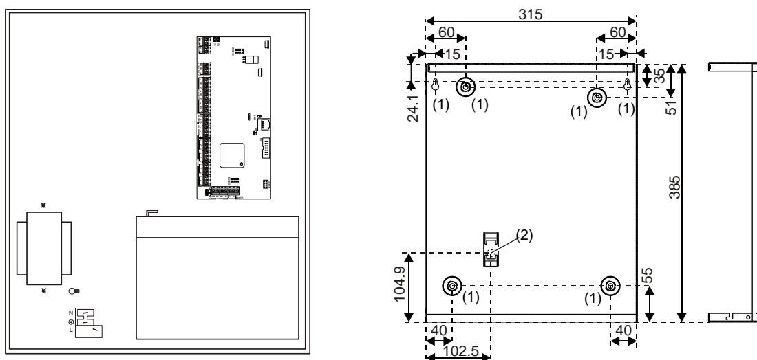
Figuur 2: Medium metalen behuizing (-MM)
