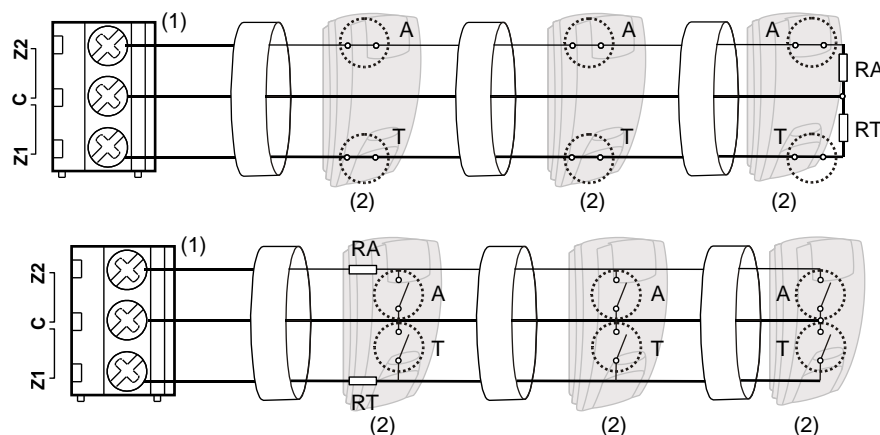
Figuur 15: Voorbeelden van enkelvoudige lus
