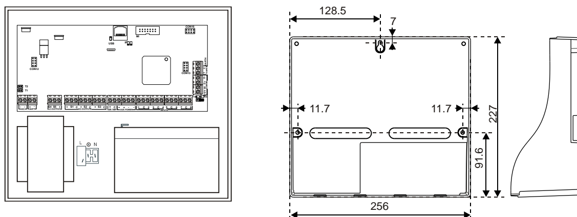
Figuur 4: Kleine kunststoffen behuizing (-SP)
