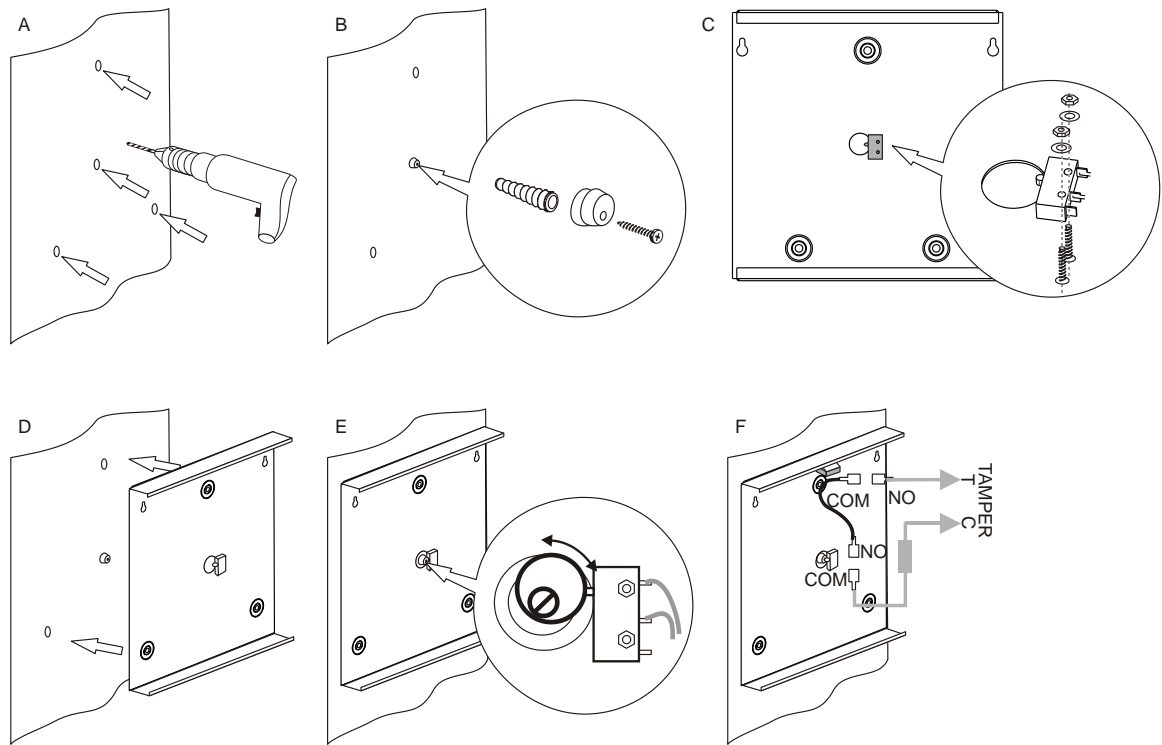
Figuur 5: Montage kleine (-SM) behuizing afneembeveiliging
