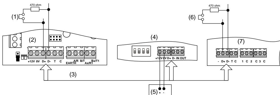
Figuur 14: Aanbevolen bedrading systeemdatabus
