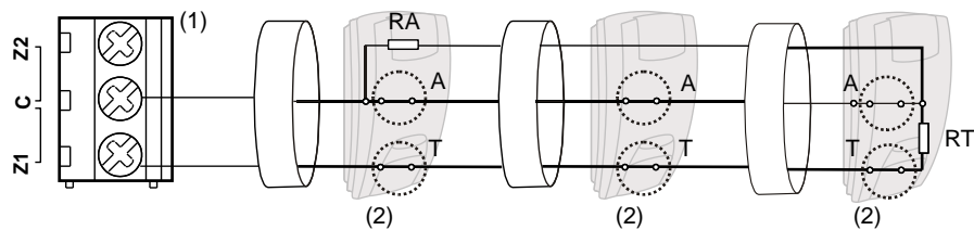
Figuur 16: Voorbeeld van Dubbellus
