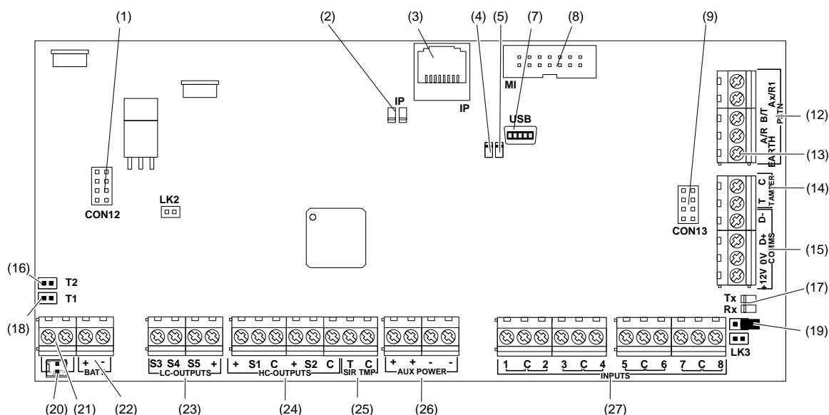
Figuur 7: Advisor Advanced ATSx000A(-IP)-aansluitschema
